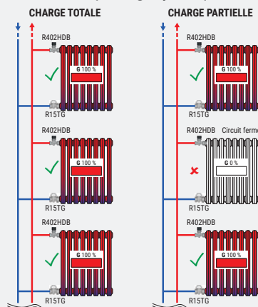
Système de colonne montante avec robinets série DB, avec équilibrage dynamique
