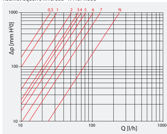
Robinet équerre inversée - R415PX033
