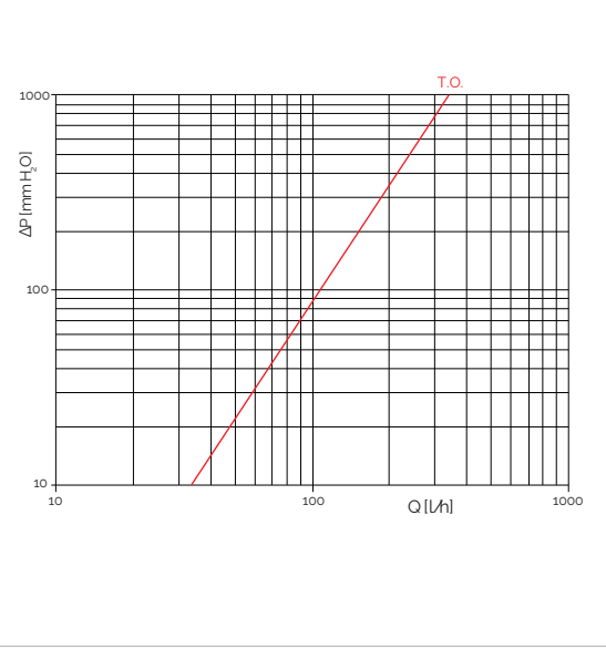
Pertes de charge R553FS
