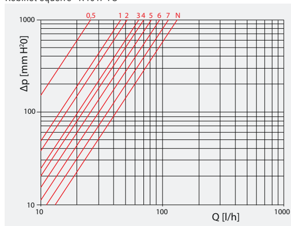
Robinet équerre - R401PTG
