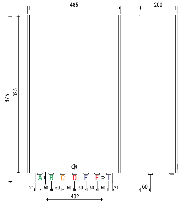
GE556-SM RADIATEUR, avec raccords par le bas, gabarit GE551Y097, isolation et coffret GE551Y194
