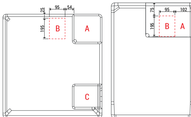
Isolation MTA version RADIATEUR Dimensions : 673x477x189 mm
